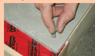
4 Trou plus grand que le diamètre de la vis
